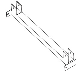
16: Haupttrahmen-Unterrohr 1 Stück
